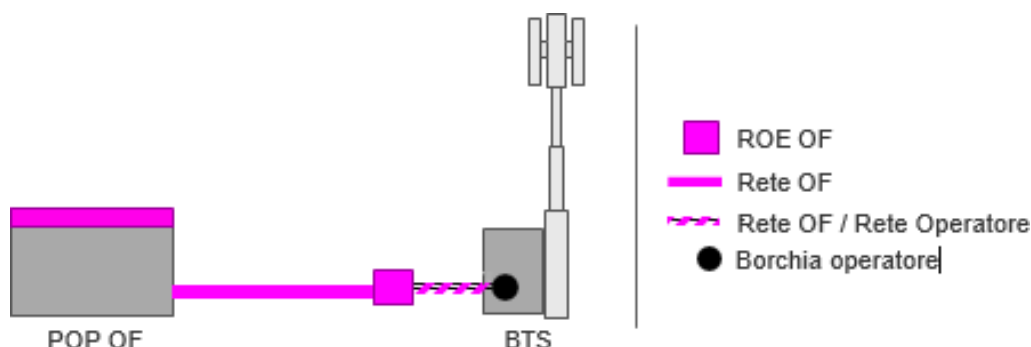
Figura 4: BTS Passiva
