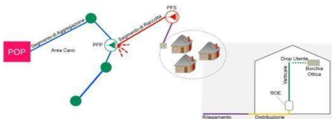
Figura 1: Esempio di architettura della Rete FTTH di OF
