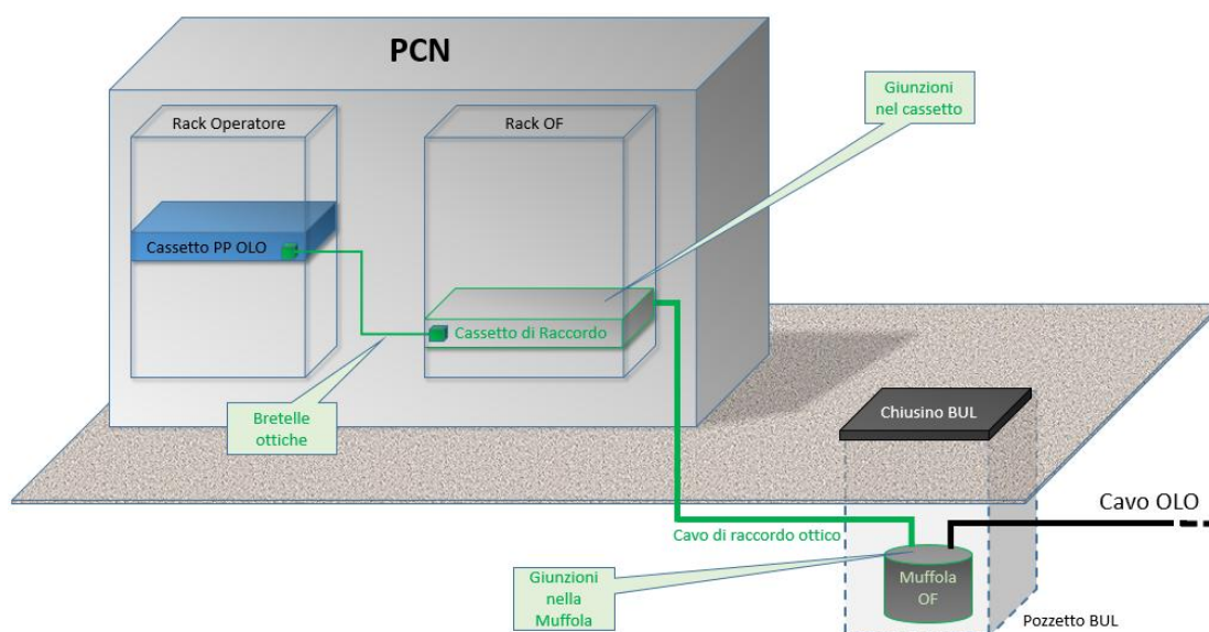
Figura 19 – Raccordo al PCN
