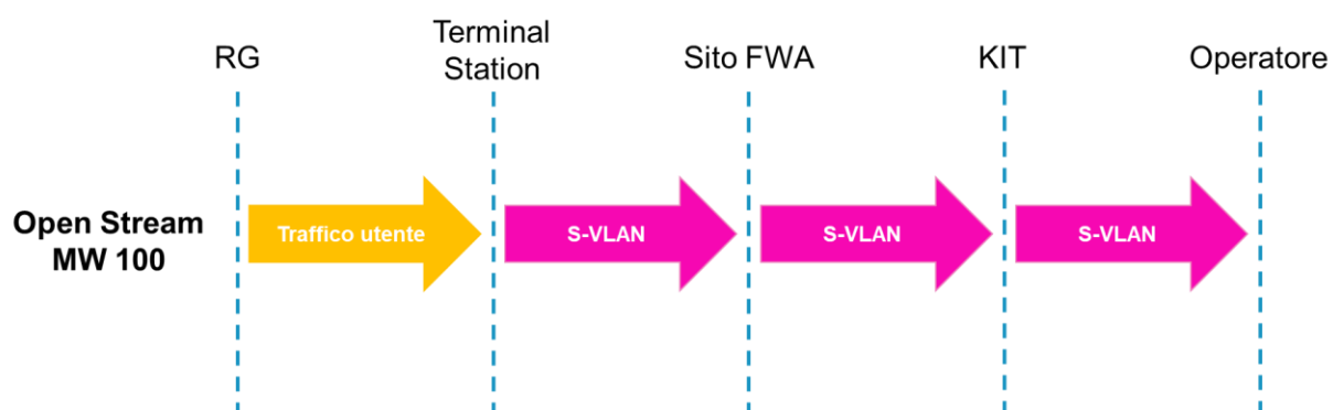
Figura 12 – Distribuzione VLAN per OpenStream MW100
