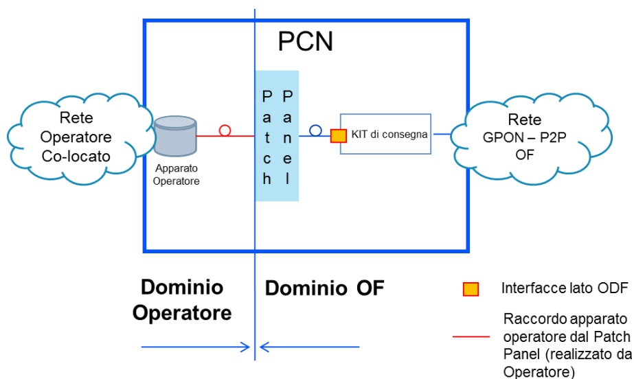
Figura 20 – Kit di Consegna e ambito di competenza OF
