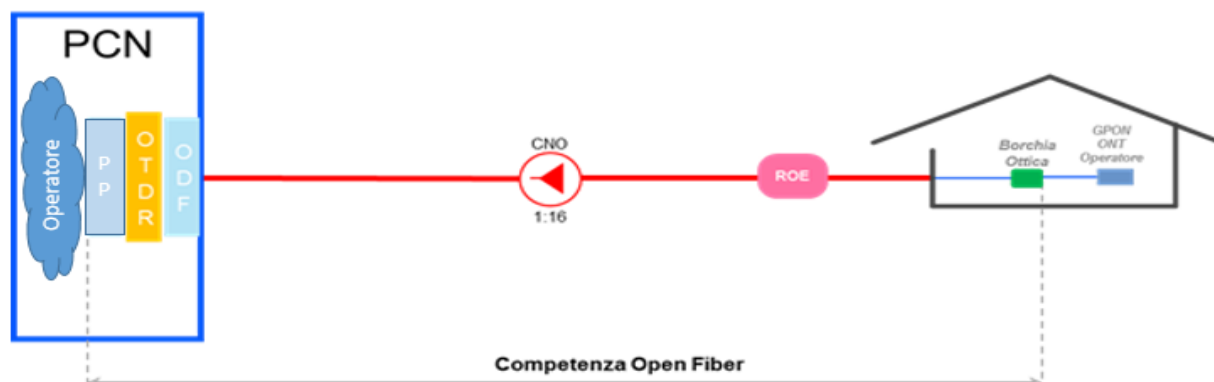
Figura 18 – Configurazione per la Colocazione al PCN
